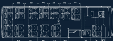
SƠ ĐỒ BỐ TRÍ GHẾ 29 CHỖ
